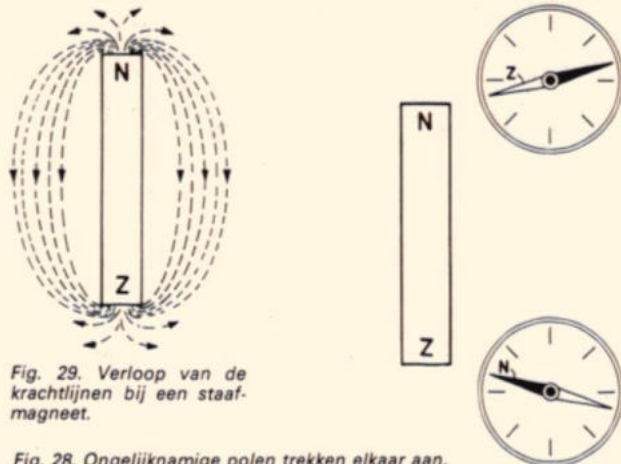
Fig. 28. Ongelijknamige polen trekken elkaar aan.
